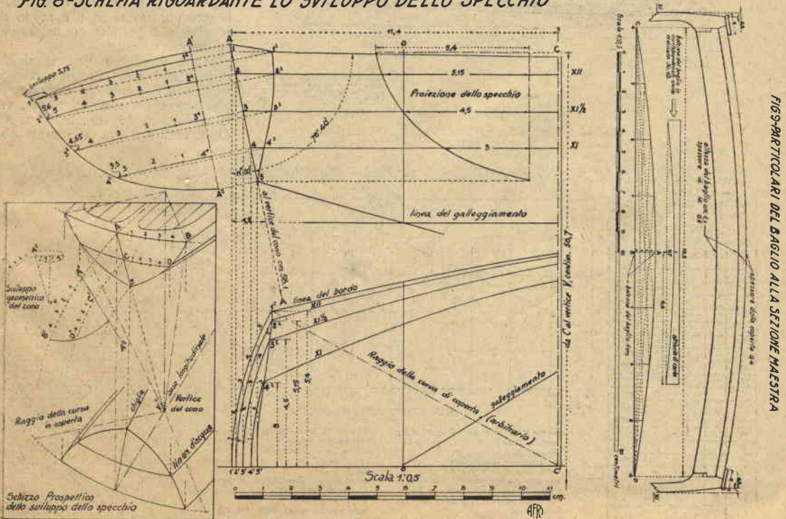
FIG.8-SCHEMA RIGUARDANTE LO SVILUPPO DELLO SPECCHIO
