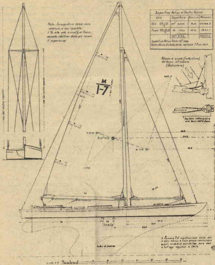
FIG.11-PIANO VELICO E CALCOLI RELATIVI
