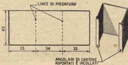
Fig. 4 - (in basso) - Involucro esterno
