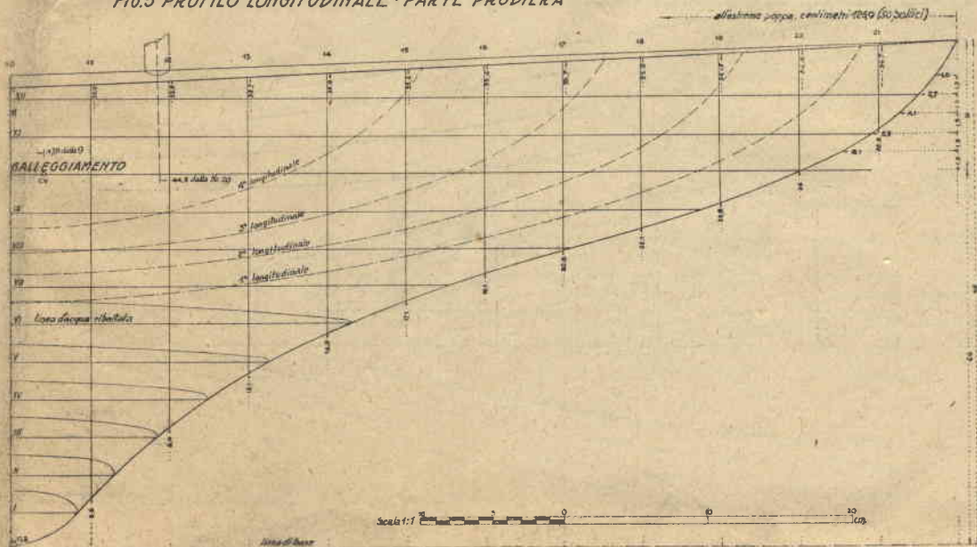
FIG. 5 - PROFILO LONGITUDINALE - PARTE PRODIERA
